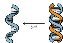
الرنا المرسل
